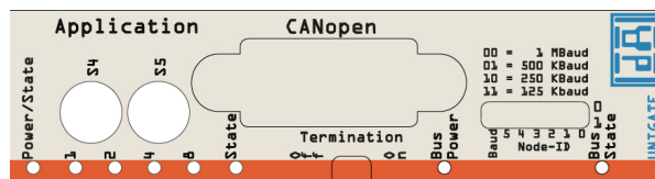
Bild 2: Frontblende: Drehschalter, DIP-Switch, Leuchtanzeigen und Terminierung CO
